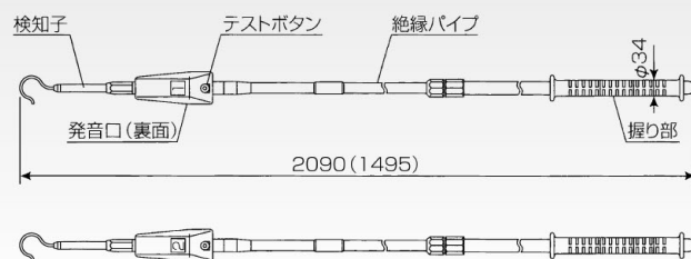
●外形寸法図(mm)
