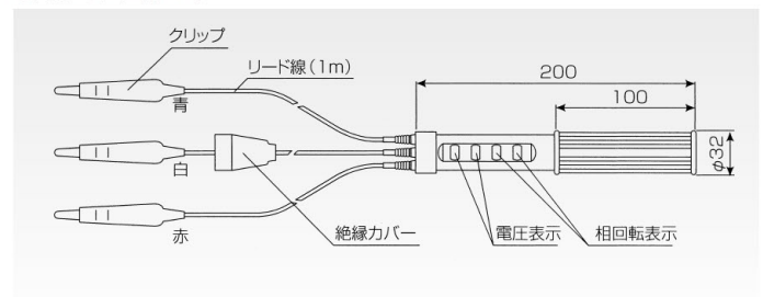
●外形寸法図(mm)
